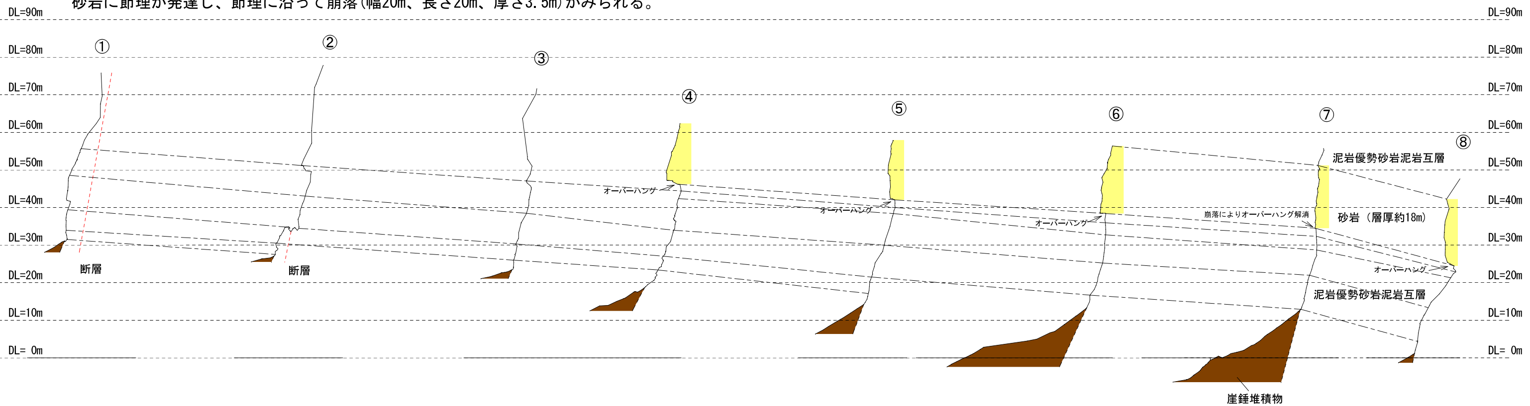
断面図 S=1:1000
