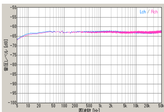
後方左右入力時レベル特性 ( 青:左チャンネル 赤:右チャンネル )
