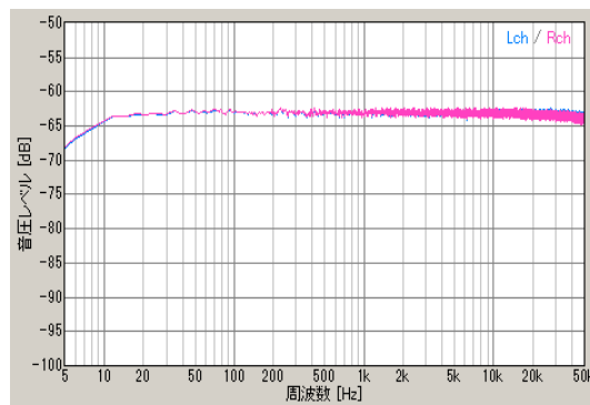
後方左右入力時レベル特性 ( 青:左チャンネル 赤:右チャンネル )
