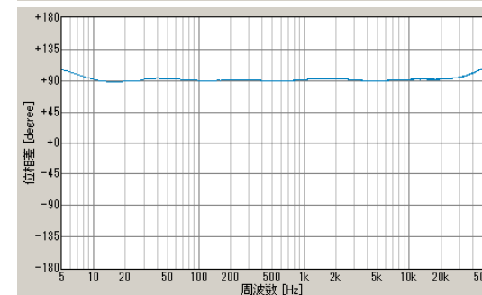
右後方入力時 位相特性
