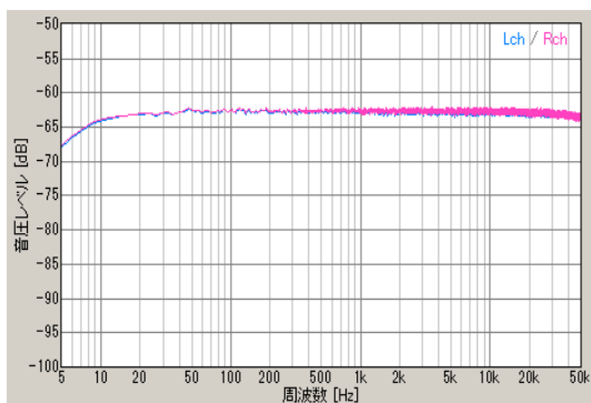
前方左右入力時レベル特性 ( 青:左チャンネル 赤:右チャンネル )
