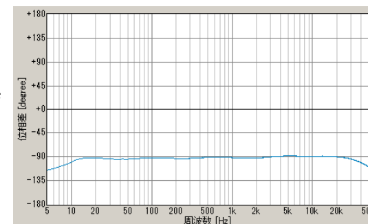
左後方入力時 位相特性
